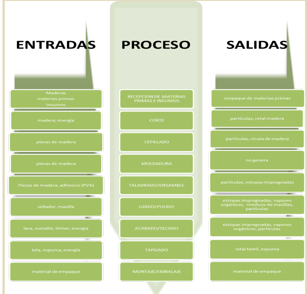
ILUSTRACIÓN No. 9. Entradas y salidas en la industria maderable - Fábricas maderables y talleres de artesanías.
